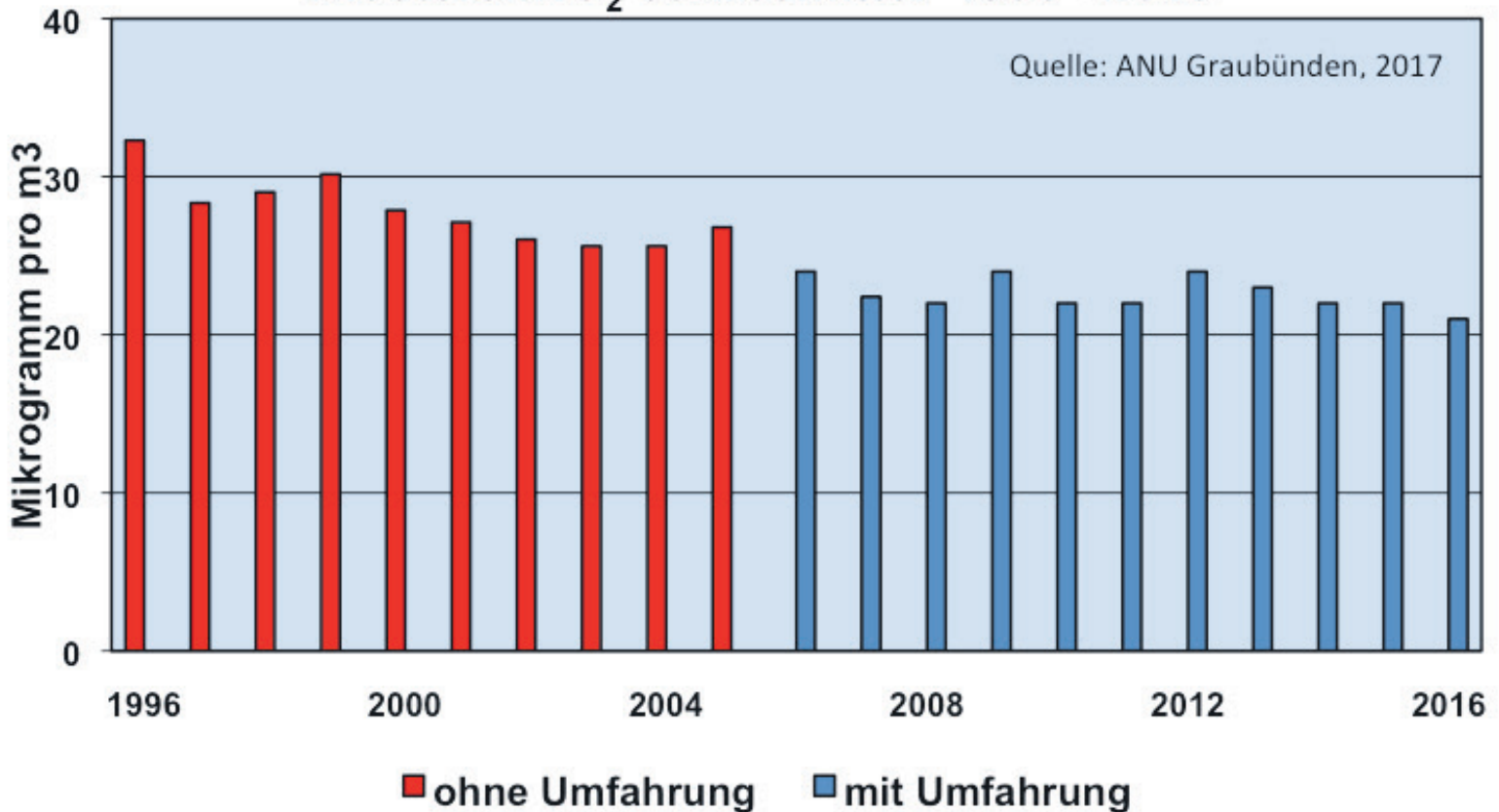
Klosters: NO 2 -Jahresmittel 1996 - 2016
