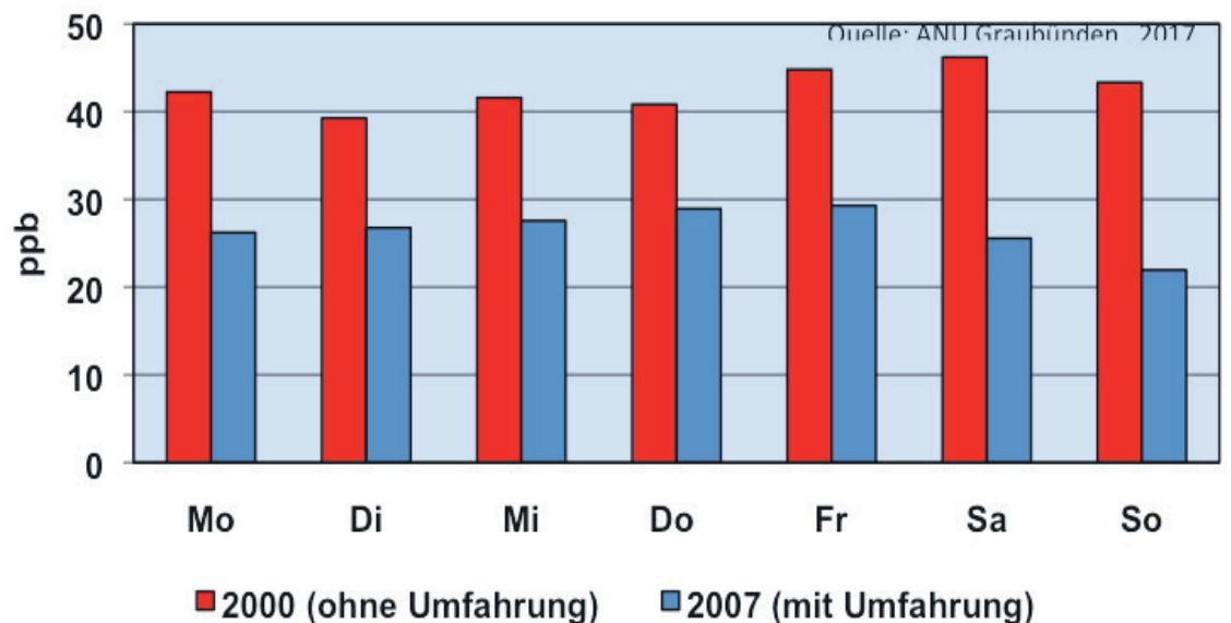
Klosters: NOx-Wochengang Januar - März
