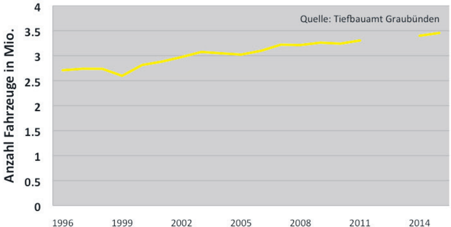
Klosters/Mezzaselva: Jährliche Verkehrsfrequenzen 1996 -2015 **
